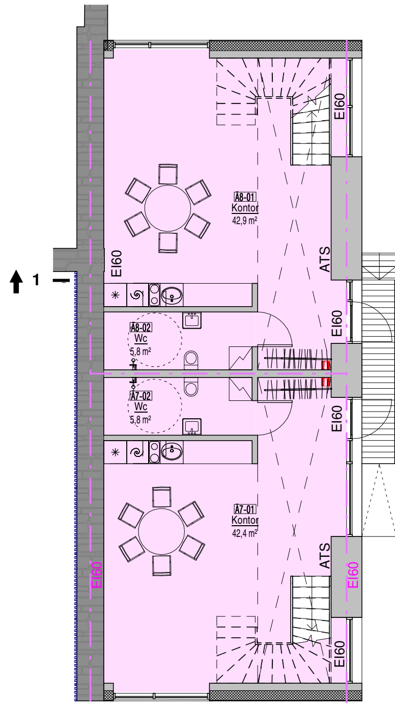
1. KORRUSE PLAAN
