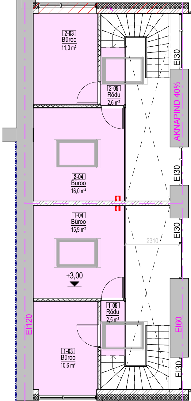
2. KORRUSE PLAAN
