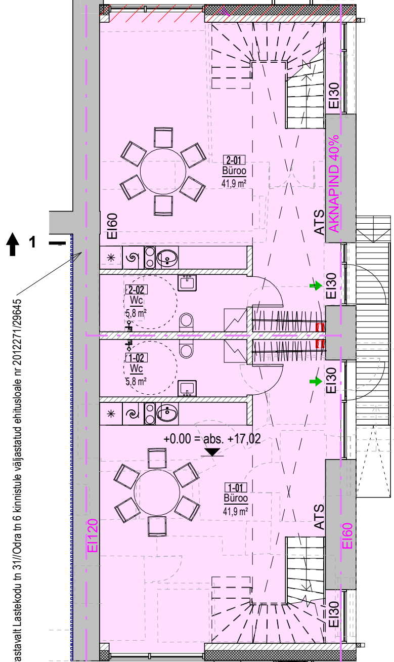
1. KORRUSE PLAAN
