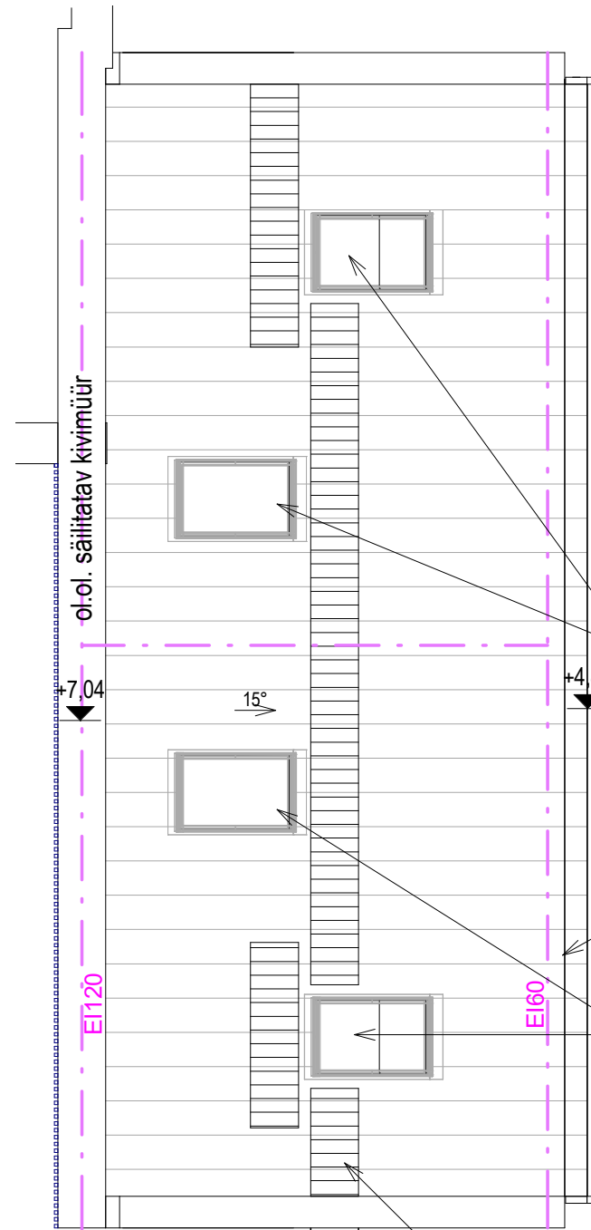
KATUSEPLAAN
